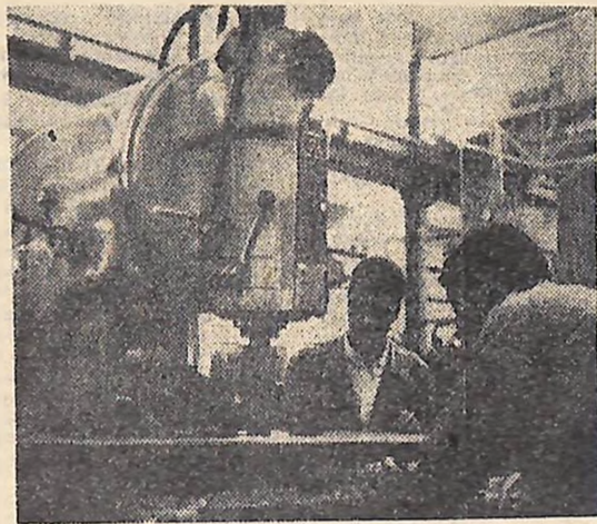
Радянський Союз надає ОАР економічну і технічну допомогу, постачає їй обладнання для різних галузей промисловості. На фото: біля пульту управління електроспечей на заводі кольорової металургії в місті Хелуані, обладнання для якого було поставлено Радянським Союзом. Фото А. ГОРЧЕВА, АПН.
