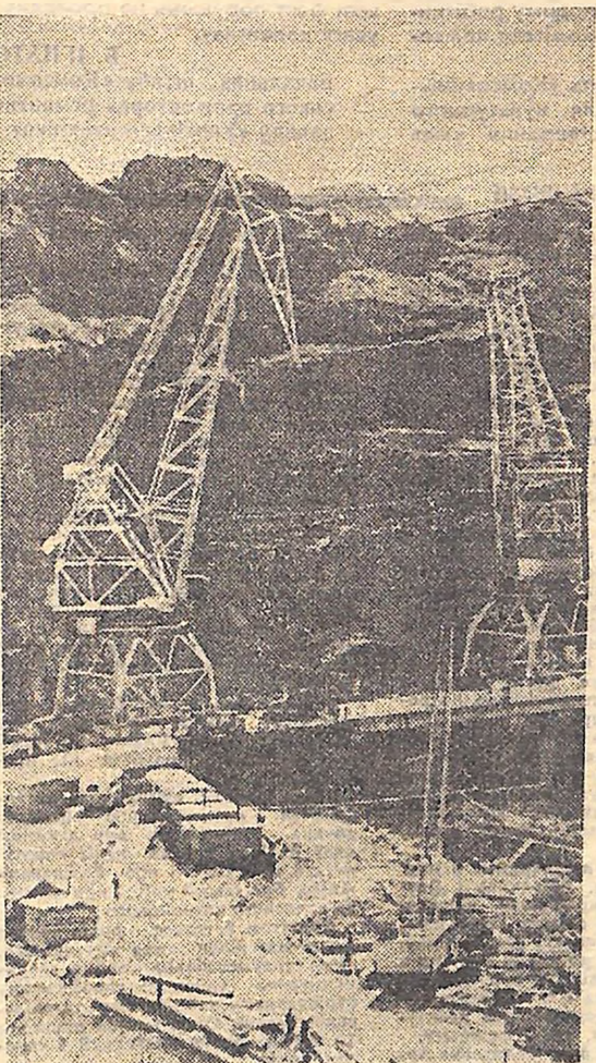
Неподалік від Алма-Ати, на річці Ілі, споруджується Капчагайська ГЕС. Чотири агрегати станції матимуть потужність 434 тисячі кіловат. Іде заповнення Капчагайського водосховища, яке протягнеться майже на 180 кілометрів. Величезна кількість води в напівпустелі дасть можливість різко збільшити виробництво рису в заснованих тут радгоспах.
