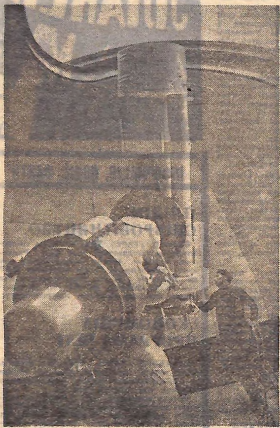
На Шемахівській астрофізичній обсерваторії, що розташована за 140 кілометрів від Баку, нещодавно почав працювати 700-міліметровий дзеркальний телескоп. Він призначений для візуального спостереження, фотографування і фотометрирування при дослідженні зірок. На знімку: новий телескоп Шемахівської обсерваторії.
