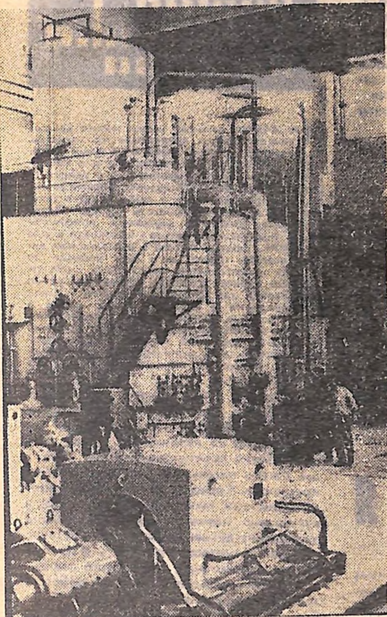
Машинний зал азотно-кисневої станції. Фото Н. ЗУБЧЕНКО.
