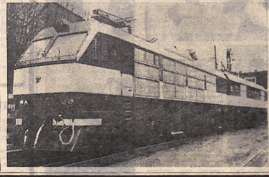
МАШИНОБУДІВНИЙ ЗАВОД «ШКОДА» В ПЛЬЗЕНІ РОЗПОЧАВ ВИПРОБУВАННЯ ЕЛЕКТРОВОЗУ З ДВИГУНОМ ПОТУЖНІСТЮ 1800 КІЛОВАТТОВИХ СИЛ. ВІН ЗРОБЛЕНИЙ НА ЗАМОВЛЕННЯ РАДЯНСЬКОГО СОЮЗУ. ДЕ ВИКОРИСТОВУВАТИМЕТЬСЯ ГОЛОВНИМ ЧИНОМ НА ЗАЛІЗНИЦІ МОСКВА — ЛЕНІНГРАД. ЕЛЕКТРОВОЗ ЗМОЖЕ РОЗВИВАТИ ШВИДКІСТЬ ДО 200 КІЛОМЕТРІВ НА ГОДИНУ. МАЄ АВТОМАТИЧНУ СИСТЕМУ УПРАВЛІННЯ, ЯКА ДІЄ ЗА ЗАДАНОЮ КОМП'ЮТЕРОМ ПРОГРАМОЮ. ЦЕ НАПІОТЪЖНІШНІЙ ЕЛЕКТРОВОЗ, ВИГОТОВЛЕНИЙ НА ЗАВОДІ ШКОДА. НА ФОТО: ЕЛЕКТРОВОЗ НОВОГО ЗРАЗКА. Фото ЧТК — АПН.
