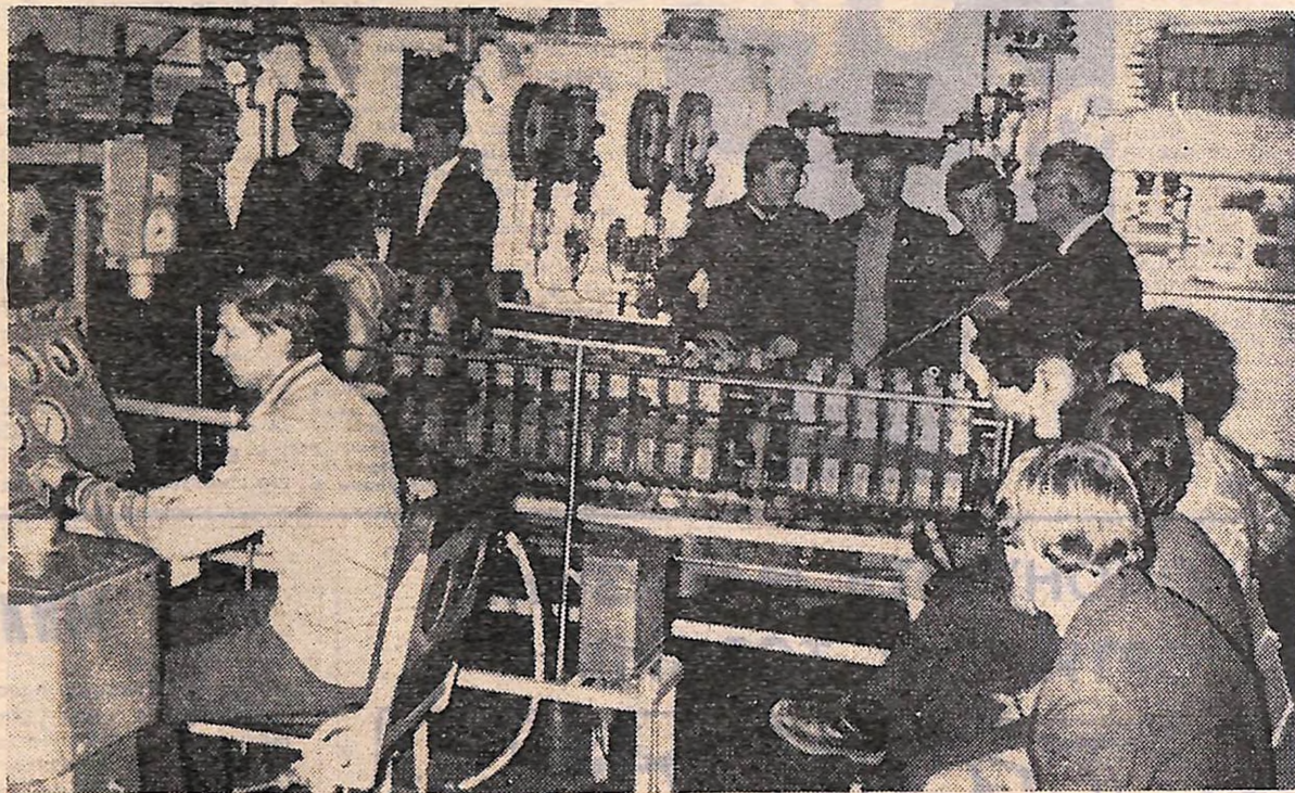
У Знамянському ТУ № 2 лабораторія по експлуатації електровозів — одна з найкращих в училищі. Обладнали її самі учні разом з викладачем Яковом Сергійовичем Гончаренком. На знімку: Я. С. ГОНЧАРЕНКО проводить додаткові заняття з групою майбутніх помічників машиністів електровозів.
