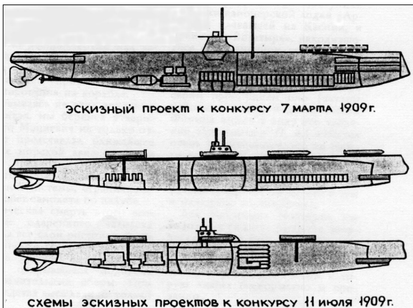
Схеми ескізнних проєктів підводних човнів, розроблених Л. М. Мацієвичем і поданих ним на конкурсі. 1909 р.
